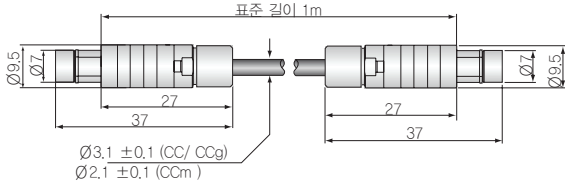
커넥터 유형 B와 센서 케이블
