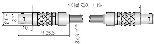
SC6000-1,0 동기화 케이블 (제품번호: 2903473)
