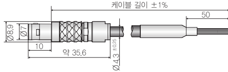
SCA3/4 신호 출력 케이블 (제품번호: 2902104)
