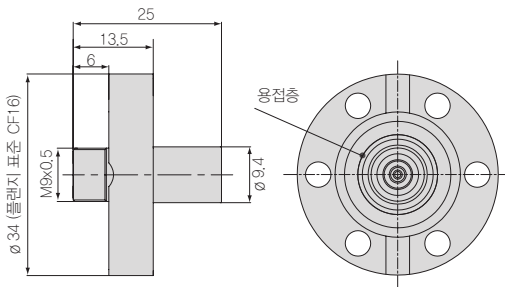
CF16 플랜지 적용 UHV/B 진공 트라이엑스 (제품번호: 0323349)
