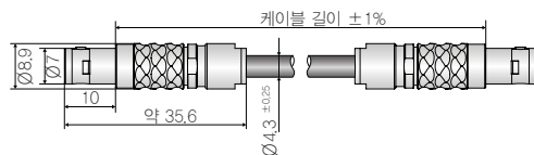
CA5 프리 앰프 케이블 (제품번호: 2903180)
