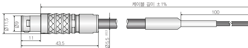
PC6200-3/4 전원-/트리거 케이블 (제품번호: 2901881)
