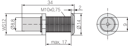
HV/B 진공 피드스쿠 (제품번호: 0323050)
