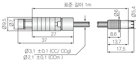
커넥터 유형 B와 센서 케이블
