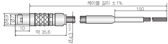
SCA3/5 신호 출력 케이블 (제품번호: 2902112)
