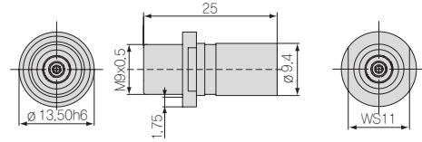
UHV/B 용접용 진공 피드 트라이엑스 (제품번호: 0323346)
