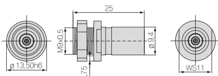
UHV/B 스크류형 진공 트라이엑스 (제품번호: 0323370)
