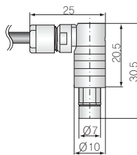
커넥터 타입 B/90
