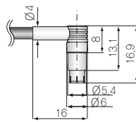
커넥터 타입 C/90
