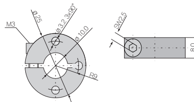
플랜지 DTA-F20
