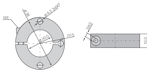
플랜지 DTA-F20
