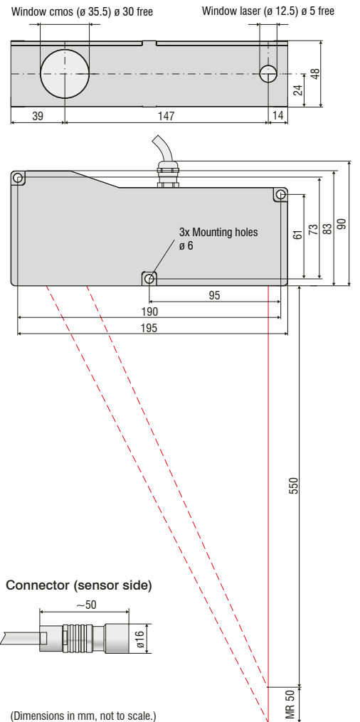
optoNCDT 2310-50
