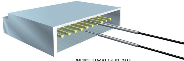
커넥팅 하우징 내 핀 검사
